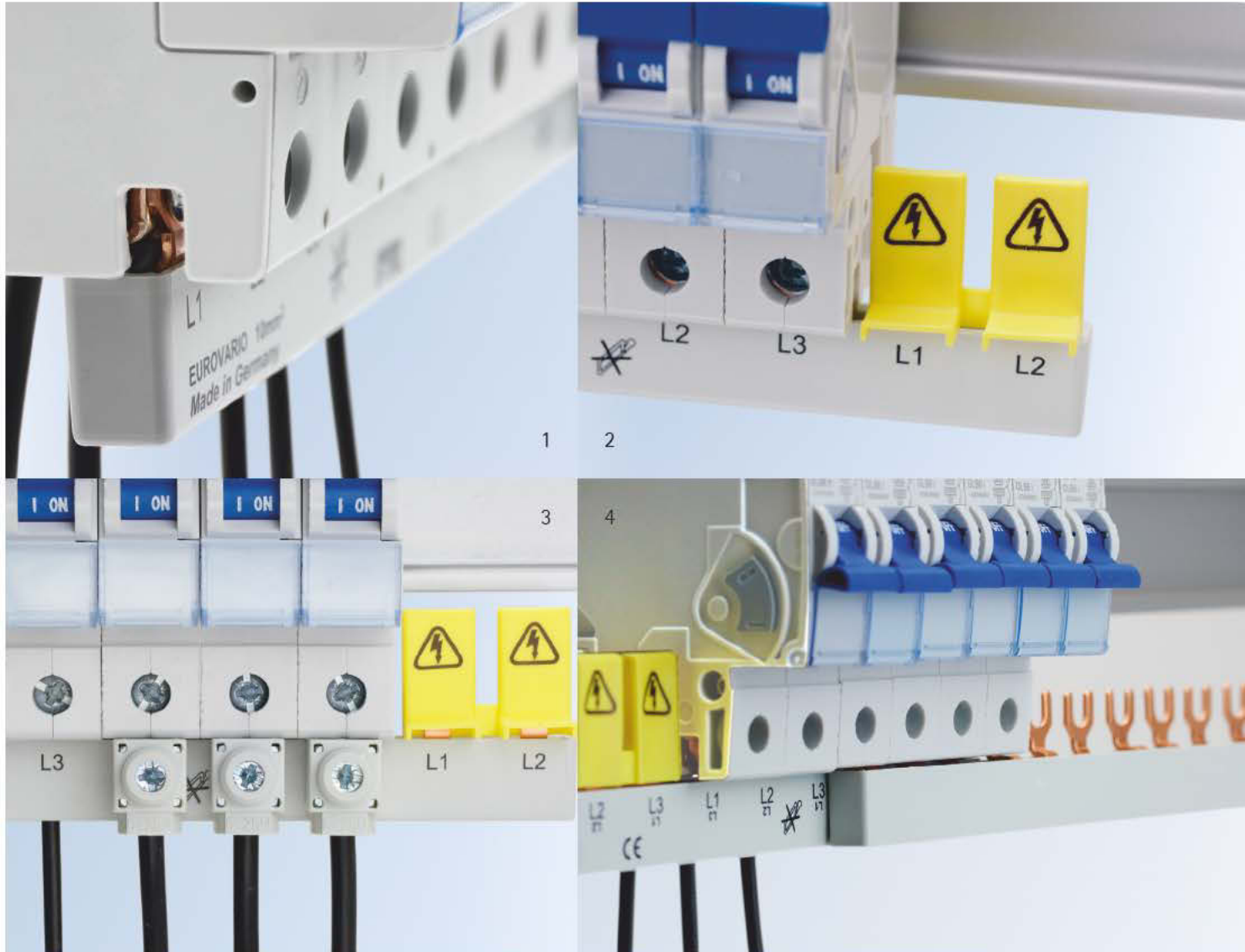
Bild 1: integrierte Endkappe | Bild 2: Berührungsschutzkappen für nicht genutzte Anschlüsse | Bild 3: Anwendung mit Einspeiseklemmen | Bild 4: Weiterverbindung von mehreren Eurovario-Schienen
